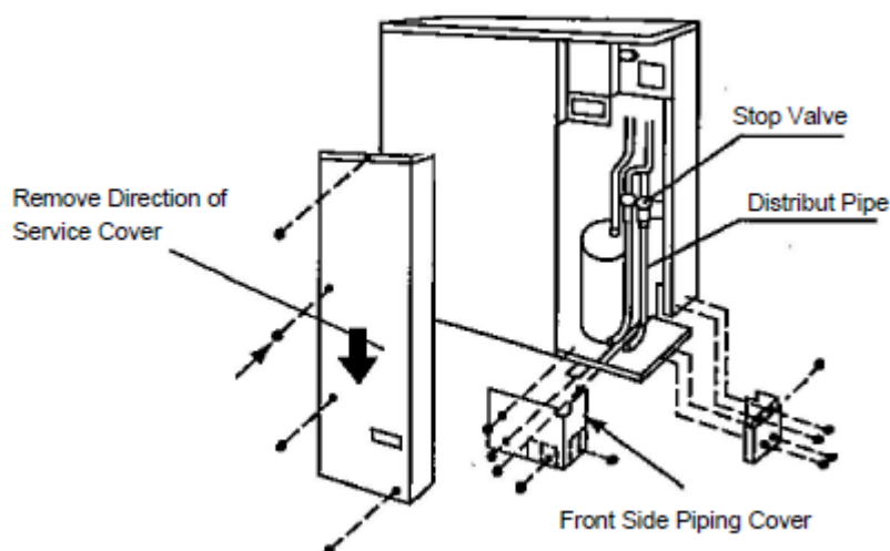
Рис.5.1 Направление трубопроводов
