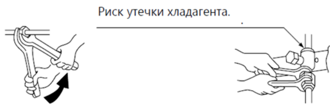
Использование двух гаечных разводных ключей Риск утечки хладагента. Затяжка запорного клапана (на линии жидкого хладагента)
