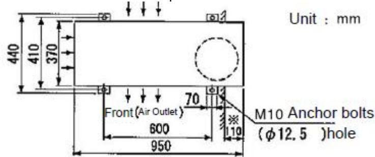
Рис. 4.3.b Положение анкерных болтов
