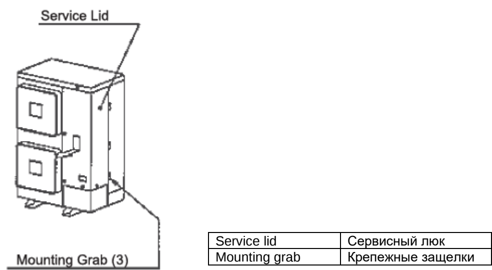
Рис. 5.2. Монтаж и удаление сервисного люка
