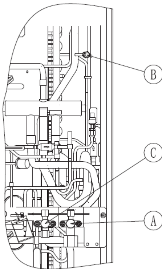
Рис.5.4 (б) Положение контрольной муфты (3 ФАЗЫ)
