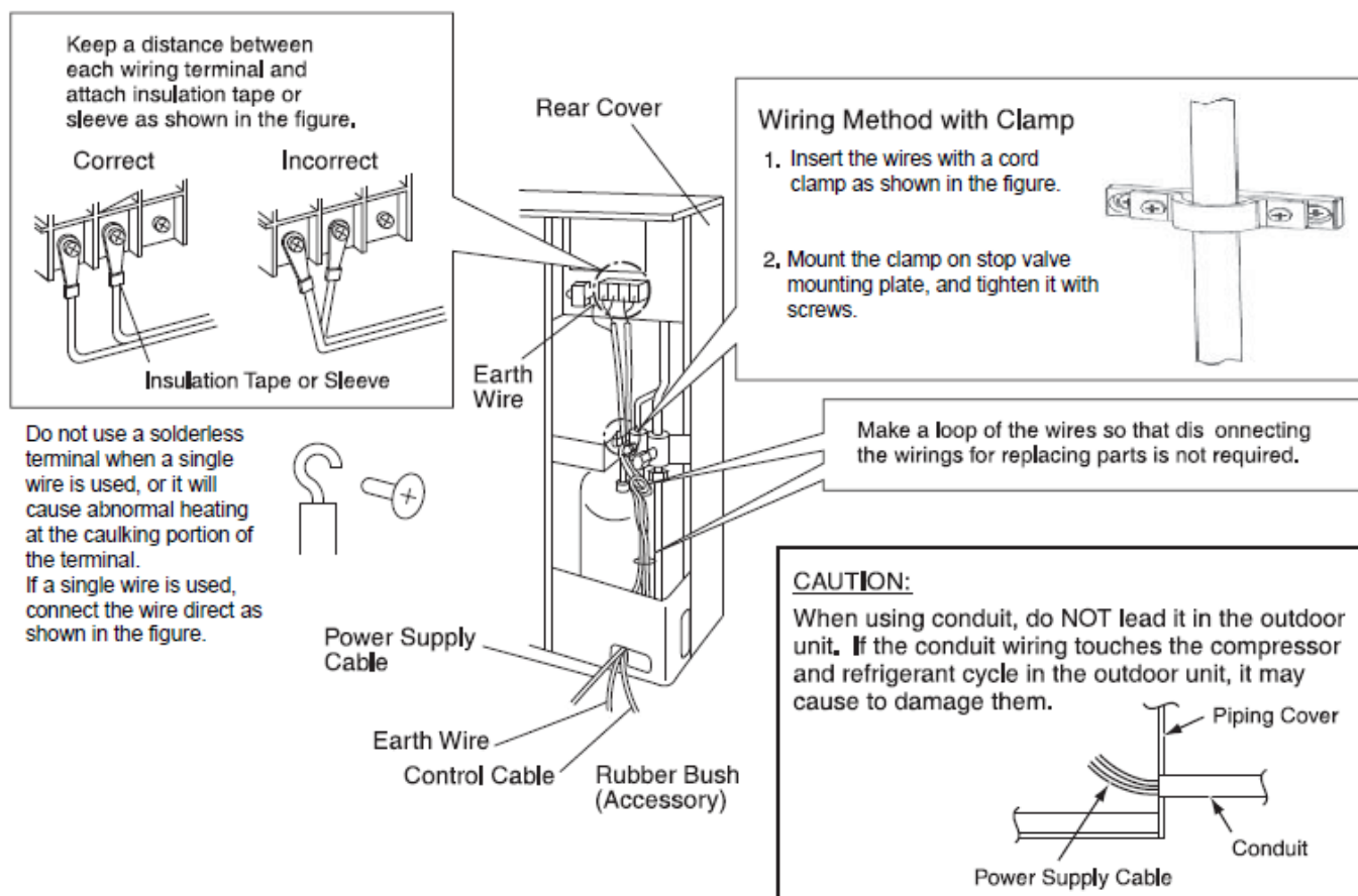
Рис. 6.3 Монтаж электропроводки для наружного блока
