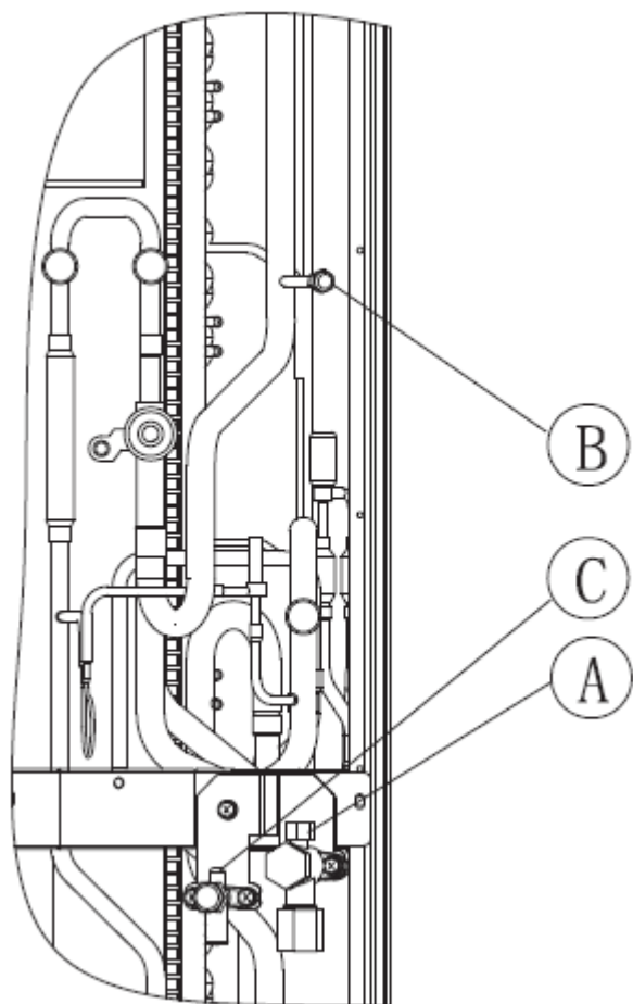
Рис.5.4 (а) Положение контрольной муфты (1 ФАЗА)
